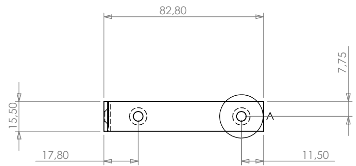
DETALHE A
